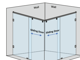
2 fixed glass & 2 sliding door
